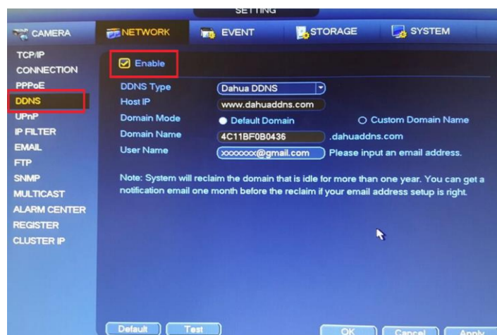
Primer pristupnih podataka putem DDNS servera
